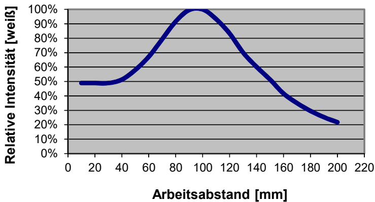
KL-M18-XL-A2.0 (fokussiert auf 200 mm) + R-S-A2.0-(2.5)-1200-67° INT [relativ]
